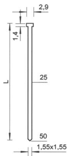
typ SKAM 400
