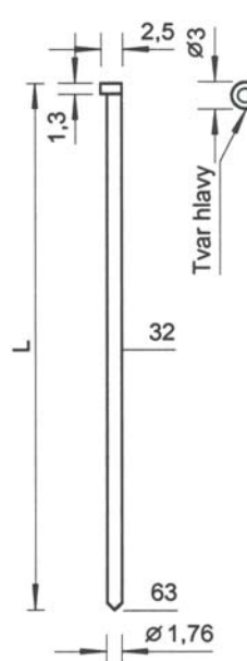
typ SKDA
