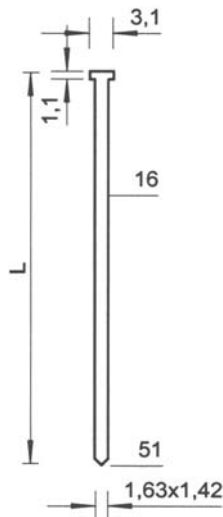
typ SK 400
