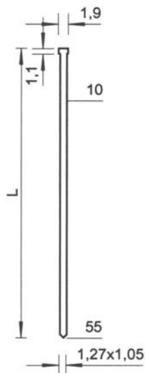
typ SKAM 400
