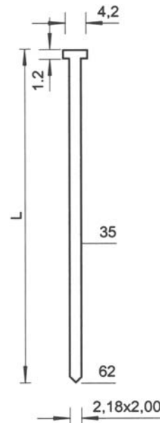
typ RSK 500
