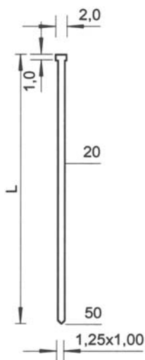
typ SKAM 300
