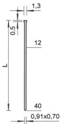
typ SK 200
